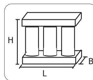
Dimensioni massime filtri riduzione dV/dt
