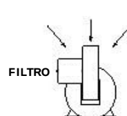
VENTILATORE A COCLEA CON FILTRO Cochlear ventilator with filter Ventilateur radial avec filter Ventilador centrifugo con filtro Schneckenlüfter mit Filter IP 23
