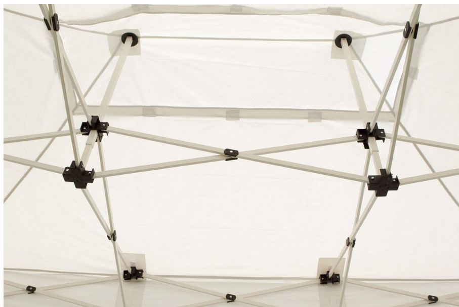
2. Sistema interno di tensionamento del tetto
