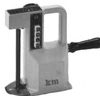
A5000KH - 200 segnatracce a caldo – altezza utile mm 200 temperature da 300 a 500° monofase 220V
