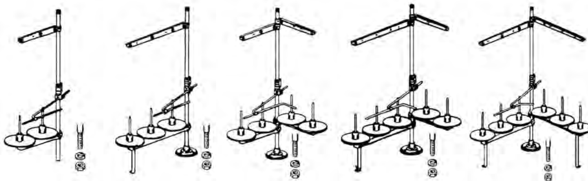
K2 K3 K4 K5 K6 Portaspole con passafilo superiore , in metallo verniciato BEIGE - versione identica al modello Mauser / W&G
