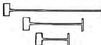
A3002 fili naylon standard (S) A3002FINE fili naylon fini (X) misure disponibili mm. standard: 15,20,25,40,45,50,65,70,75,130 fine: 7,11,15,20,25,45,50,65,75 (fili colorati a richiesta)
