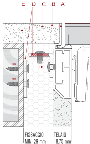
DETTAGLIO SISTEMA SPACEWALL CARTONGESSO
