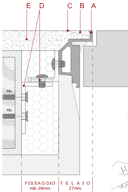
DETTAGLIO SISTEMA OPENWALL MURATURA MONTAGGIO WD A SPINGERE
