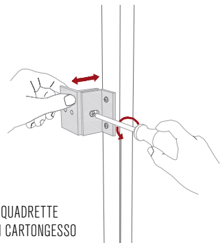
INDICAZIONE DI MONTAGGIO
