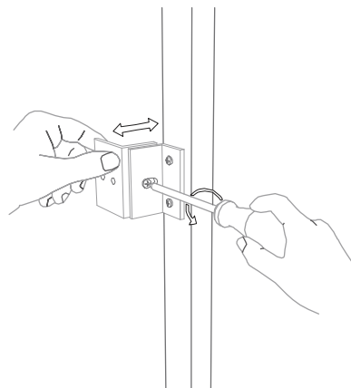
FISSAGGIO SQUADRETTE AL TELAIO IN CARTONGESSO
