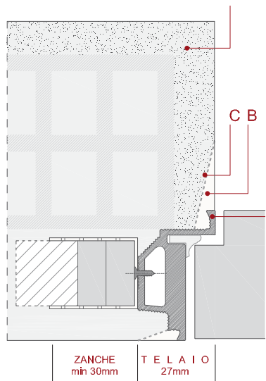
DETTAGLIO SISTEMA OPENWALL MURATURA MONTAGGIO WD A TIRARE
