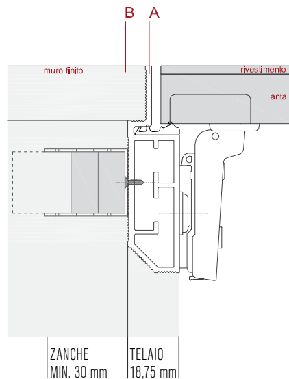
DETTAGLIO SISTEMA SPACEWALL MURATURA
