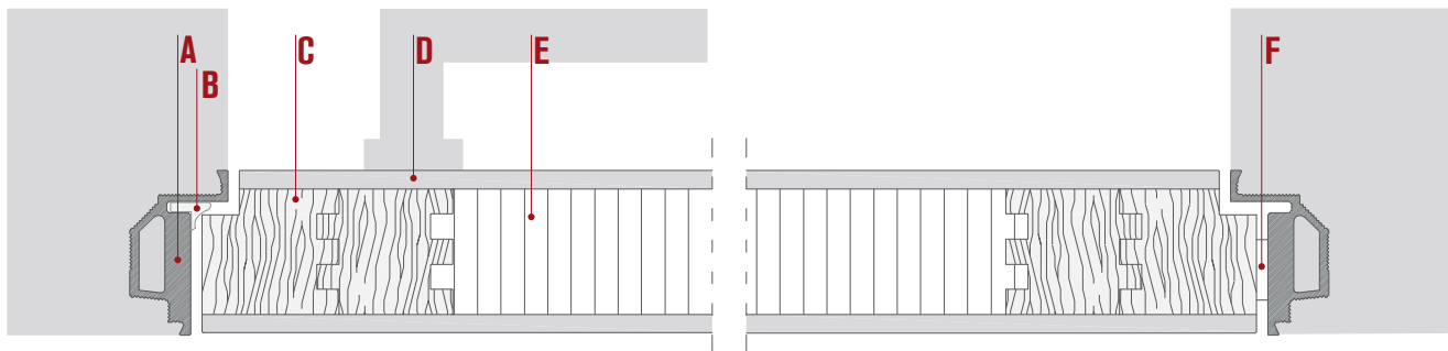
DETTAGLIO SISTEMA OPENWALL MURATURA MONTAGGIO WD A TIRARE
