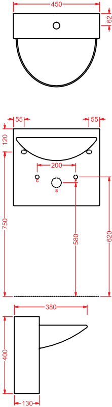
WLL001 WALL MINI lavabo sospeso wall-hung washbasin
