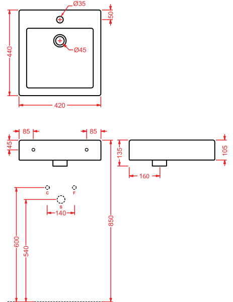
TFL017 FUORI CLASSE lavabo sospeso/appoggio 45 wall-hung/countertop washbasin 45
