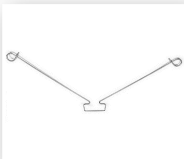
DISTANZIATORE PER PALO METALLO, CON ASTE DRITTE, SENZA GANCIO DI CHIUSURA
